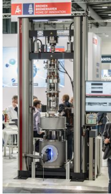
ZwickRoell Prüfanzlage HTE 2023
